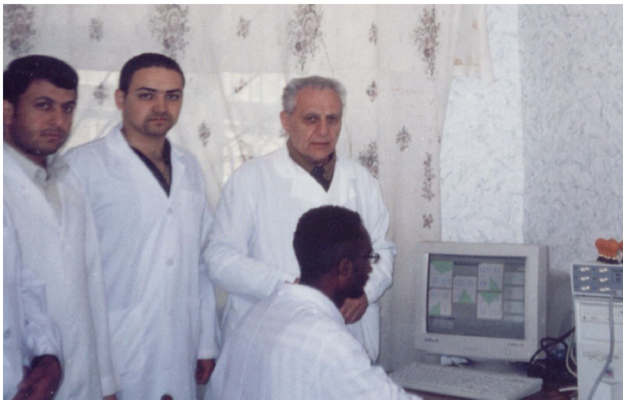
Профессор Добрин Б.Ю. знакомит иностранных студентов с изобретением кафедры – аппаратом векторэлектрокардиографом, выпущенным серийным производством Северодонецким ПО «Микротерм»
